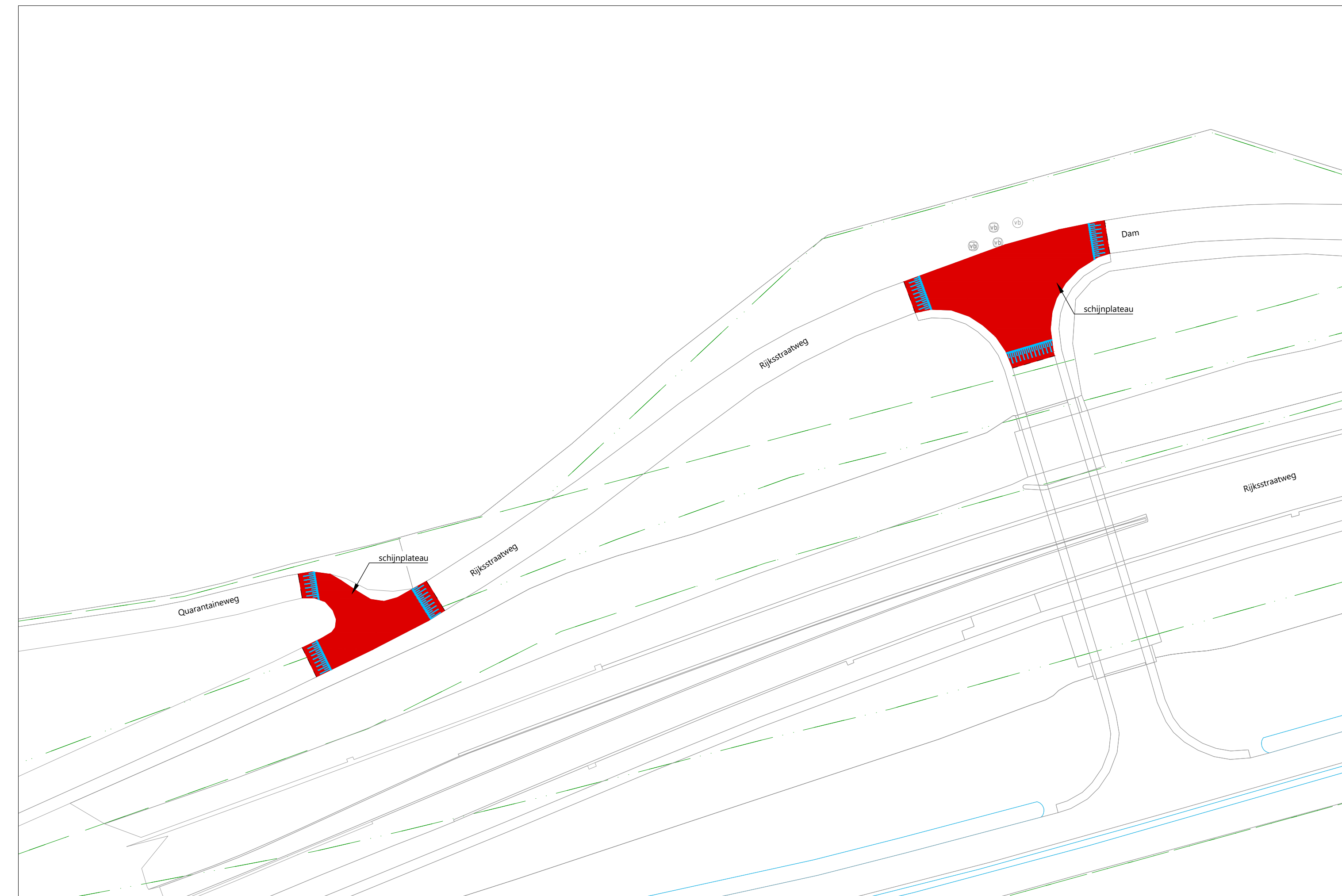
SITUATIE - KRUISSING QUARATAINEWEG - RIJKSSTRAATWEG / RIJKSTRAATWEG - DAM Schaal 1:500
