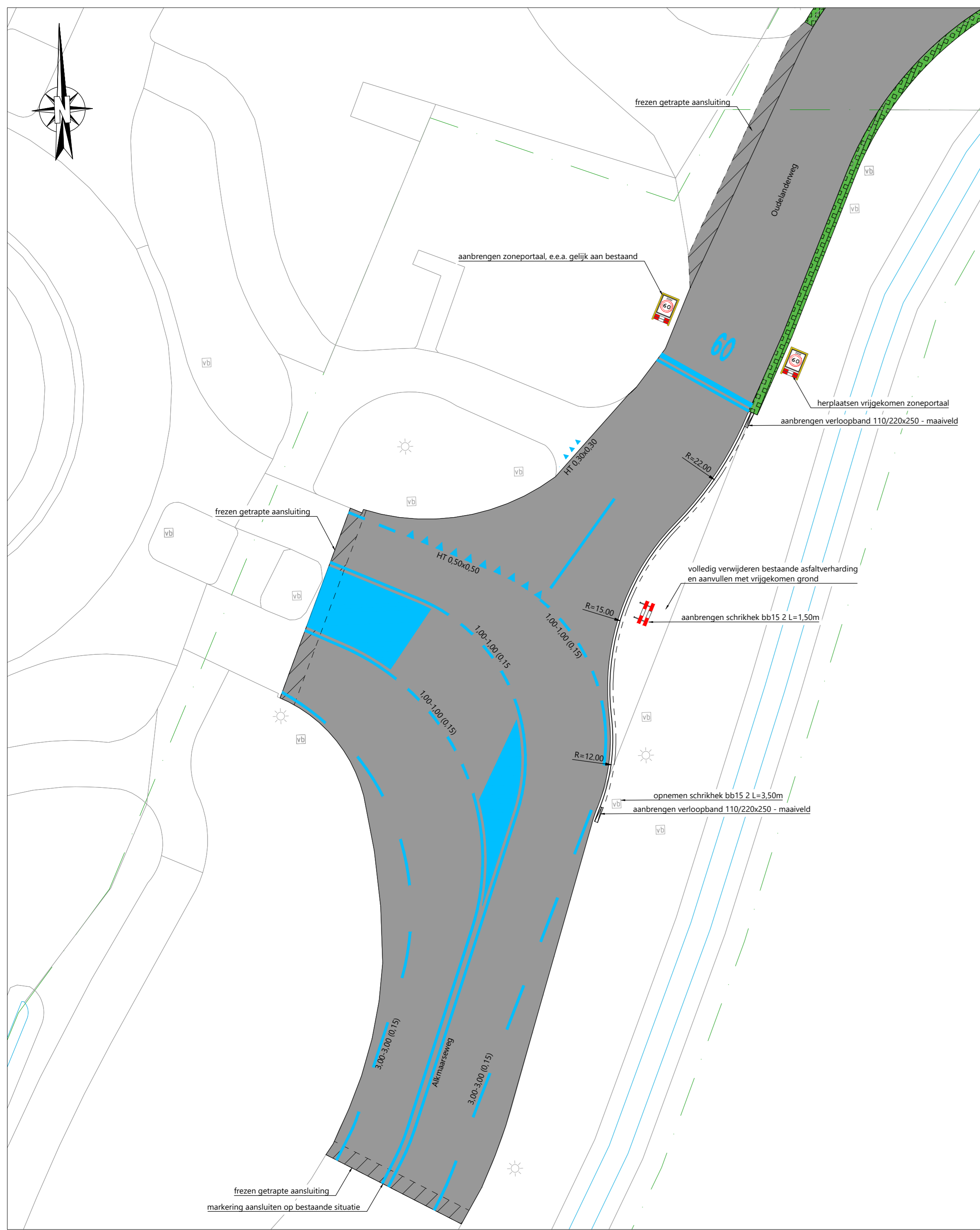
DETAIL KRUISPUNT Schaal 1:200
