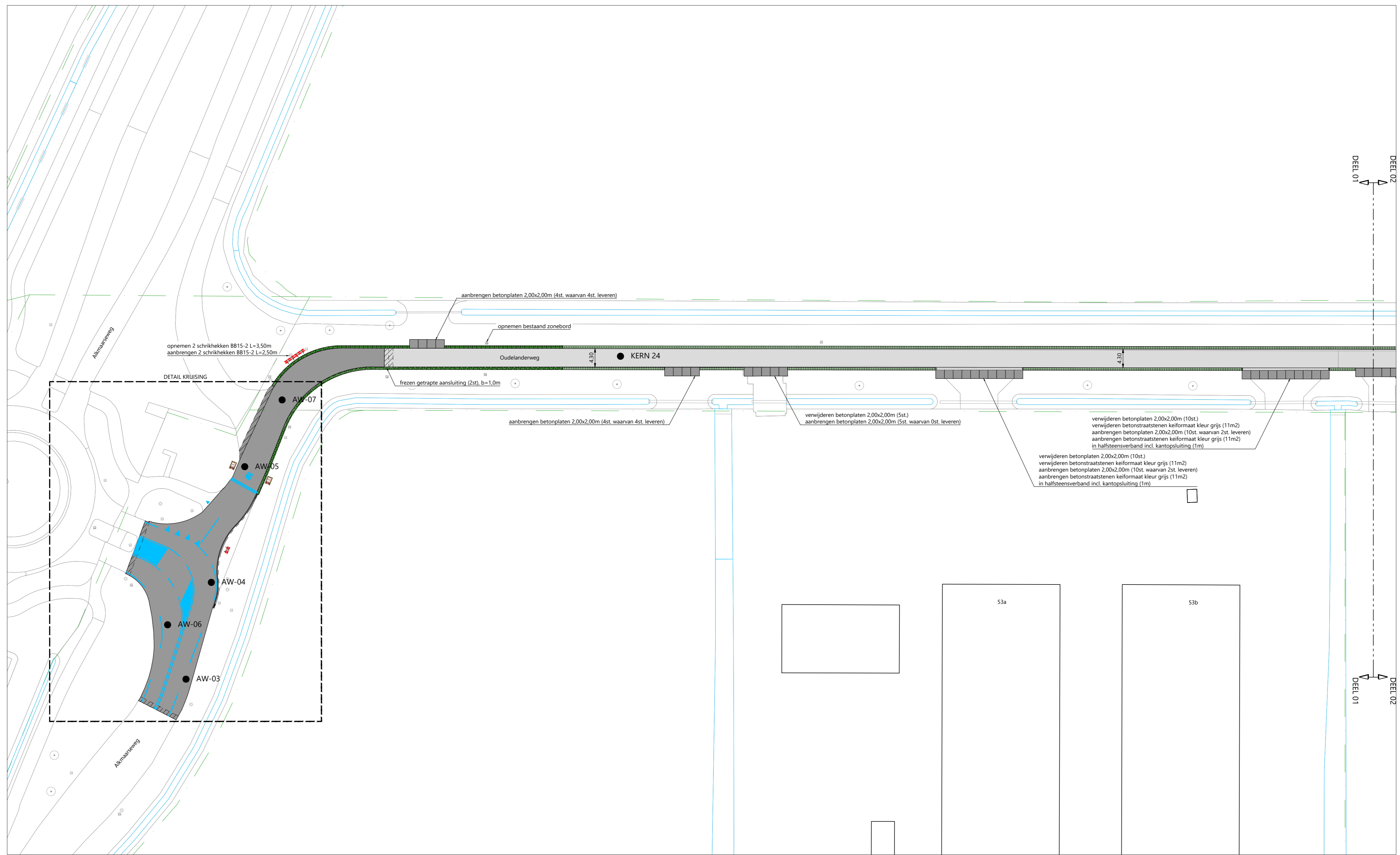
SITUATIE - DEEL 01 Schaal 1:500
