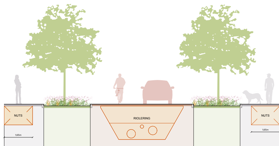
Principeprofiel hoofdinfrastructuur
