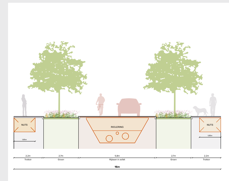
Profiel hoofdinfrastructuur zoals vastgesteld in de Nota van Uitgangspunten
