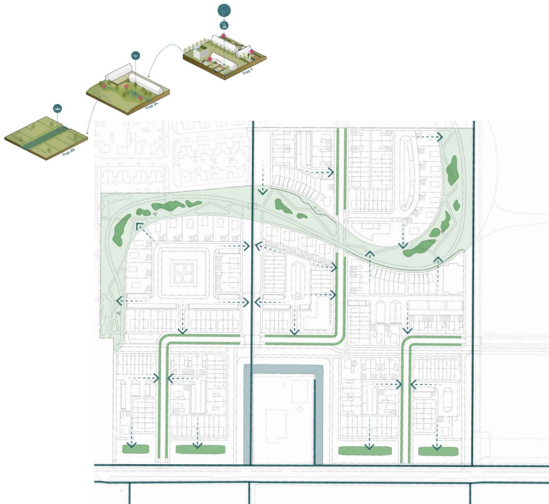
Voorbeeldverkaveling (indicatieve invulling)
